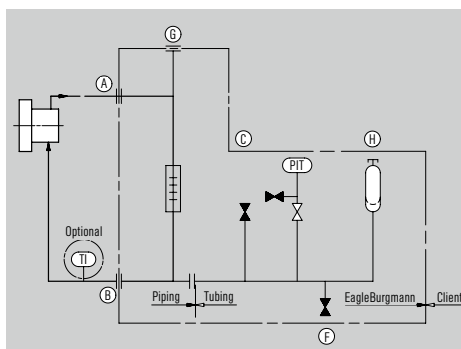
Funktions- und Installationsschema SPO, Plan 53B
